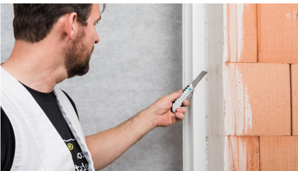
3. Dämmstoff abschneiden
